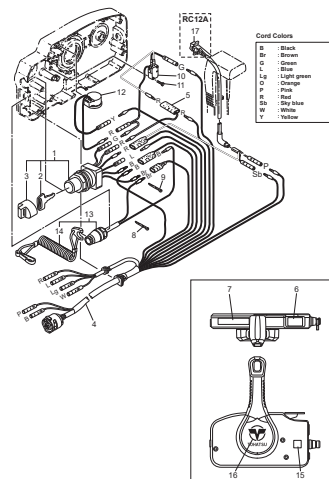
Fig.23B OPTIONAL PARTS (3) オプションパーツ (3)
