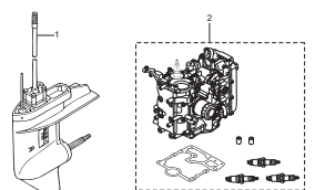
Fig. 24 ASSEMBLY • KIT PARTS アッセンブリ・キットパーツ
